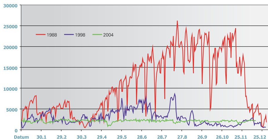
Jahresgänge der Chloridkonzentrationen von 1988, 1998 und 2004 in Gerstungen, Werra [mg/l]
