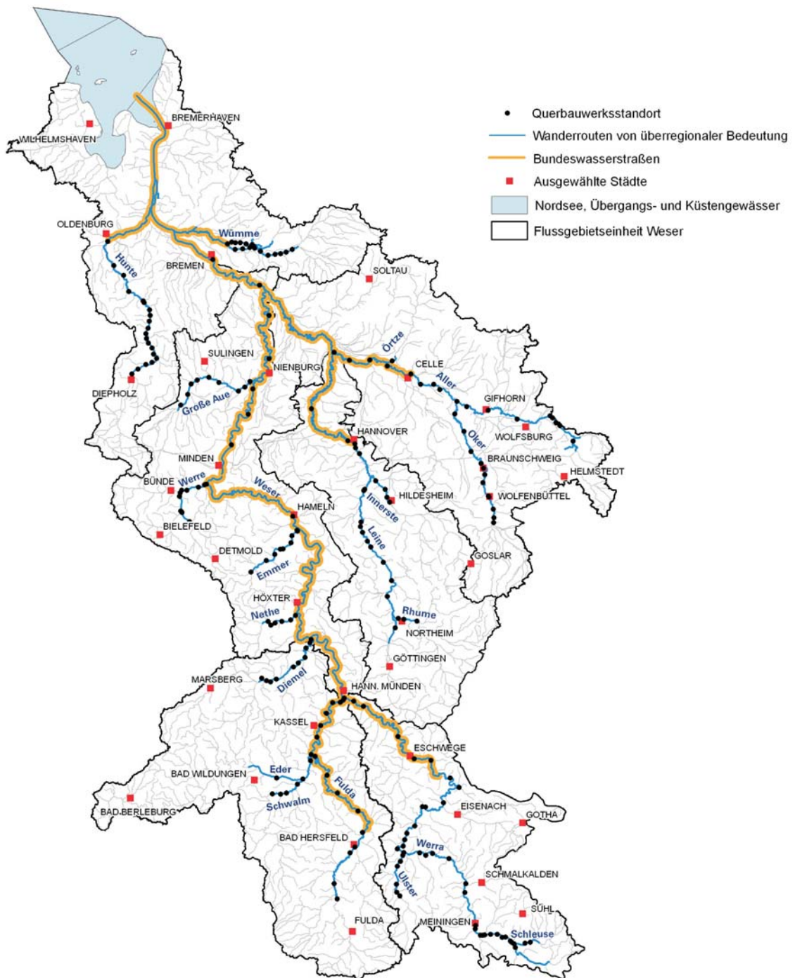
Übersicht der Querbauwerke in den Wanderrouten von überregionaler Bedeutung sowie Bundeswasserstraßen
