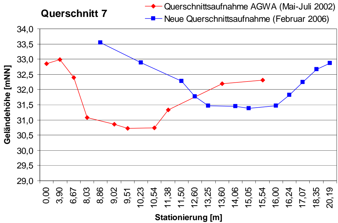
Anlage 2-7: Tiefenlage des Querschnittes 7
