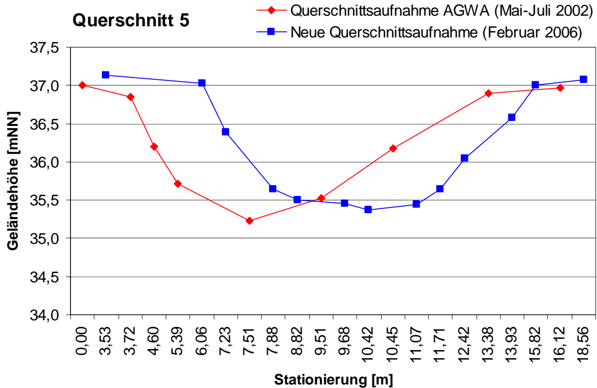
Anlage 2-5: Tiefenlage des Querschnittes 5
