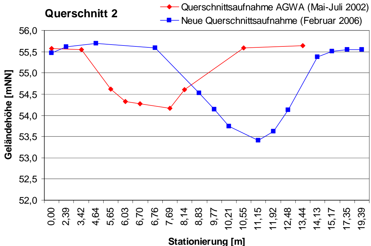
Anlage 2-2: Tiefenlage des Querschnittes 2
