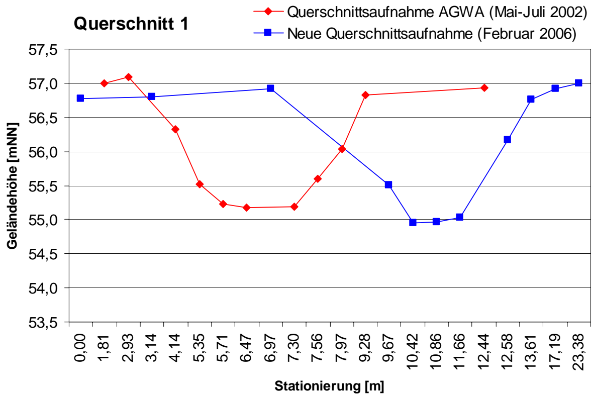
Anlage 2-1: Tiefenlage des Querschnittes 1
