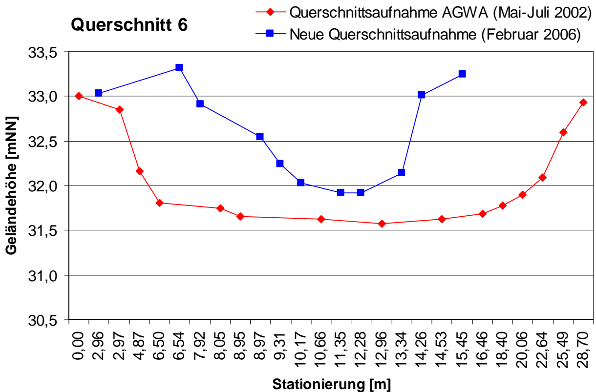
Anlage 2-6: Tiefenlage des Querschnittes 6
