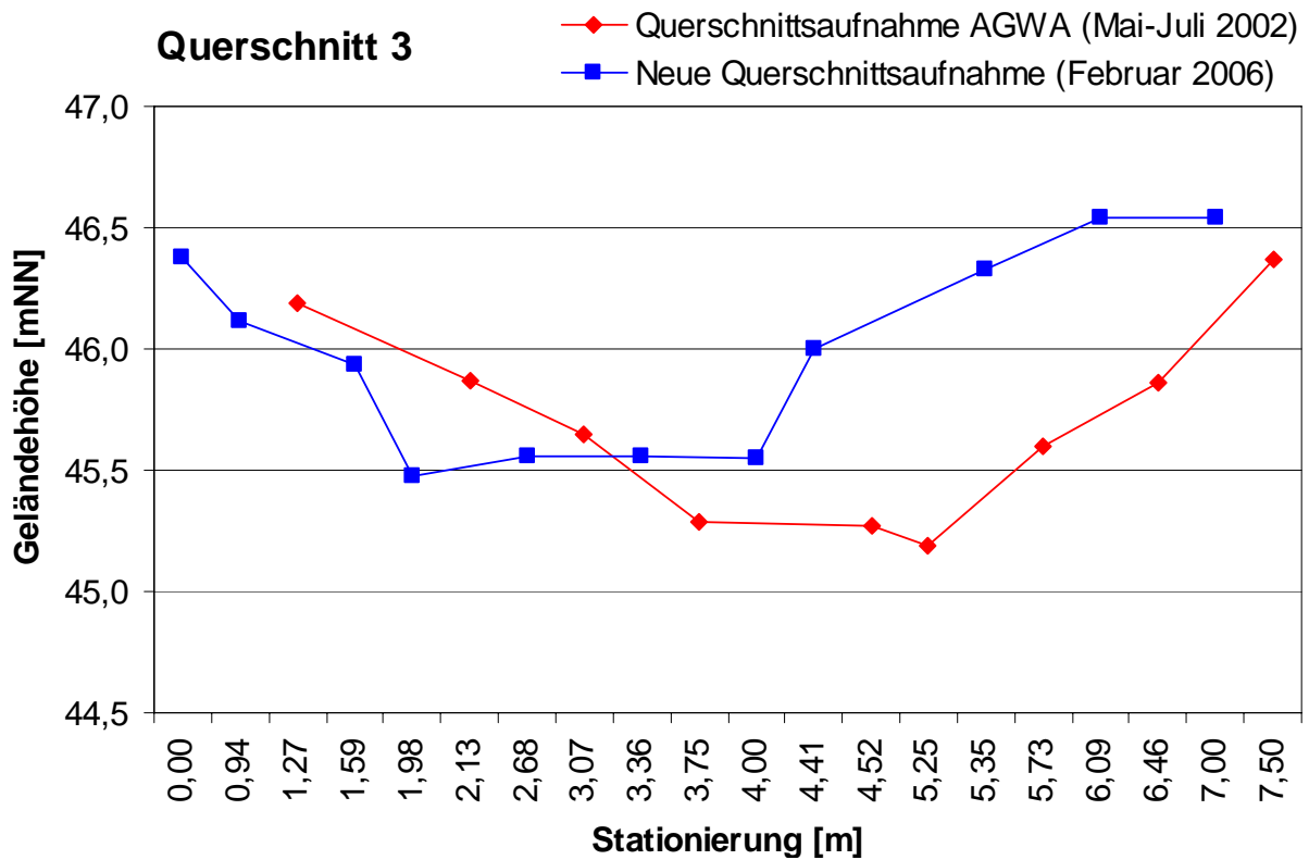
Anlage 2-3: Tiefenlage des Querschnittes 3
