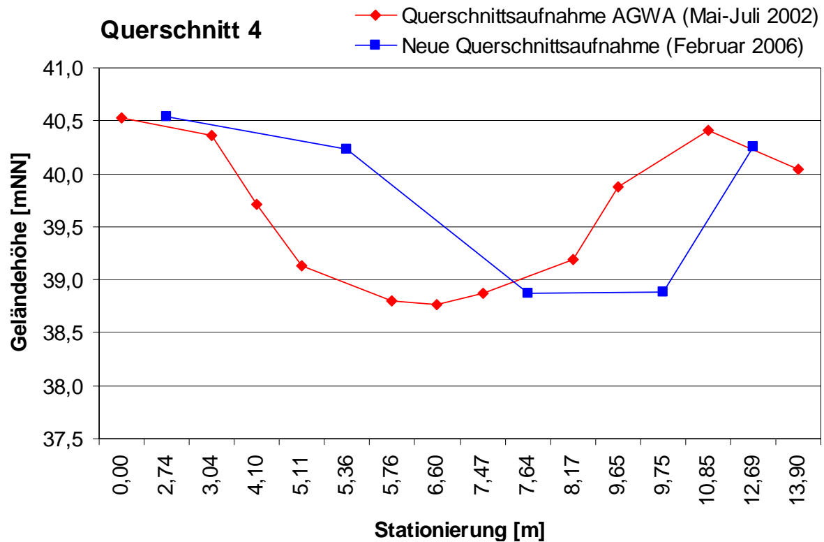
Anlage 2-4: Tiefenlage des Querschnittes 4
