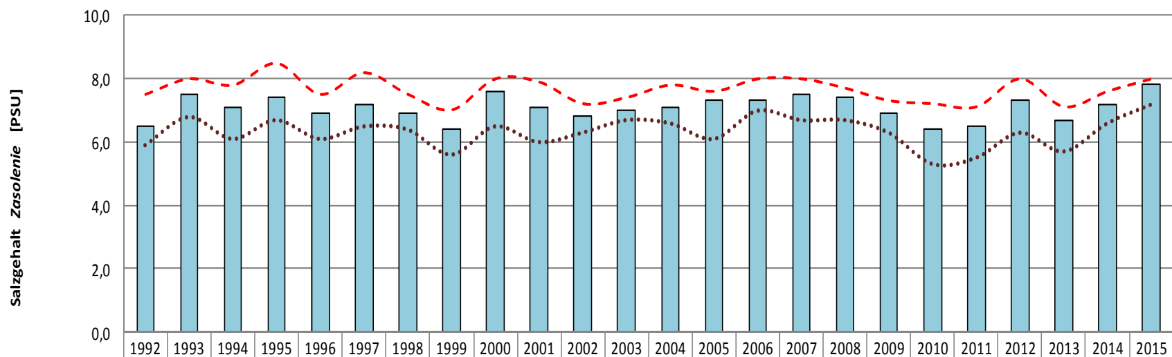
Salzgehalt (Grundnähe, April bis November), Station OB 4/IV, Pommersche Bucht, 1992 - 2015 Zasolenie (warstwa denna, kwiecień-listopad), Stanowisko OB 4/IV, Zatoka Pomorska, 1992-2015
